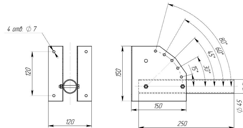
Рисунок 1. Общий вид кронштейна
