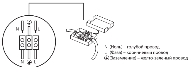
Рисунок 2. Подключение сетевых проводов
