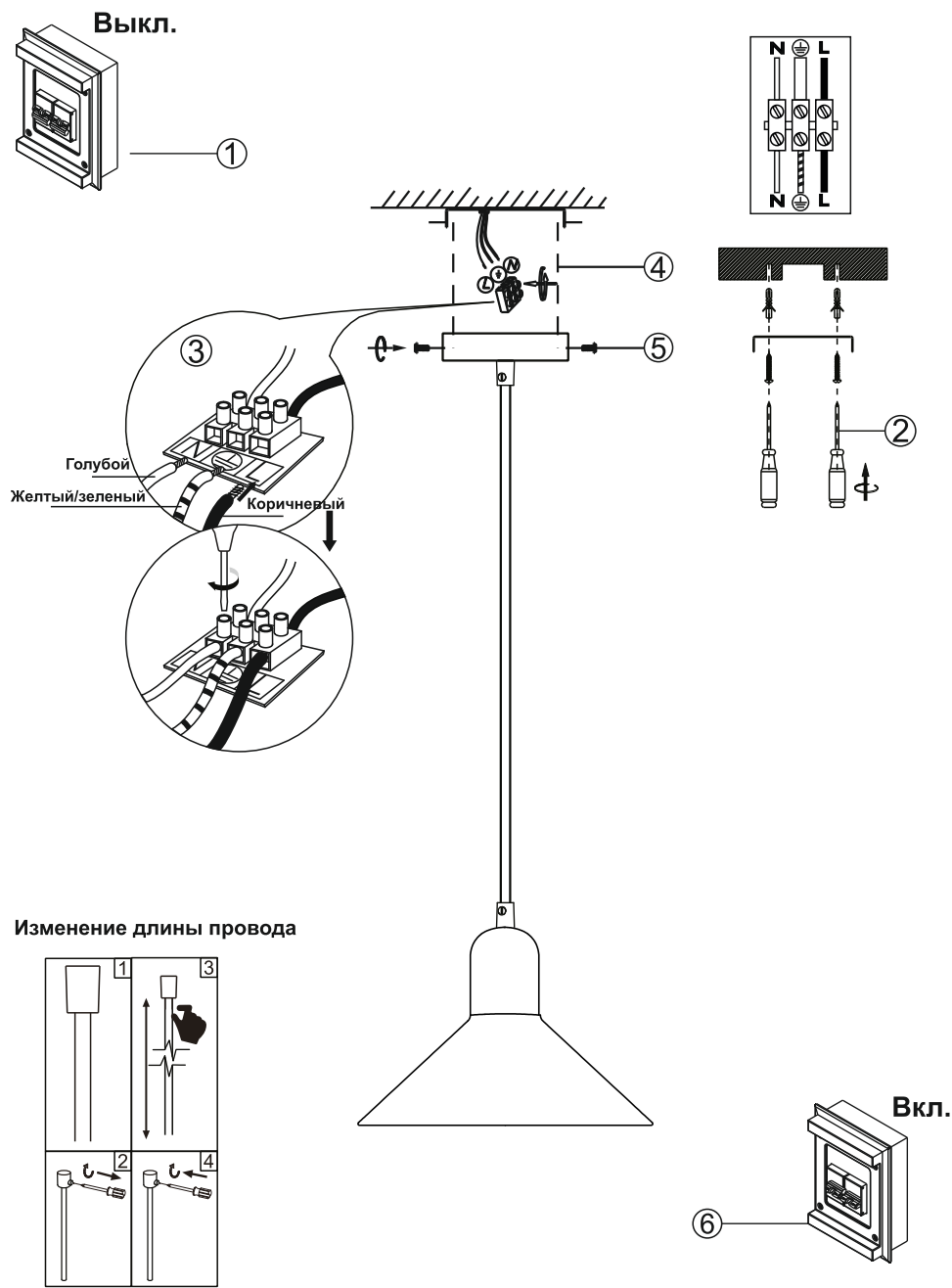
Рис.3 Установка светильника.
