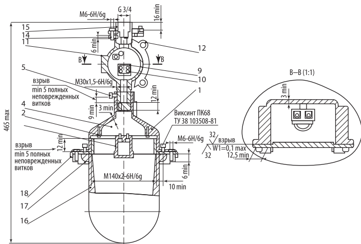
Рисунок 1. Устройство светильника
