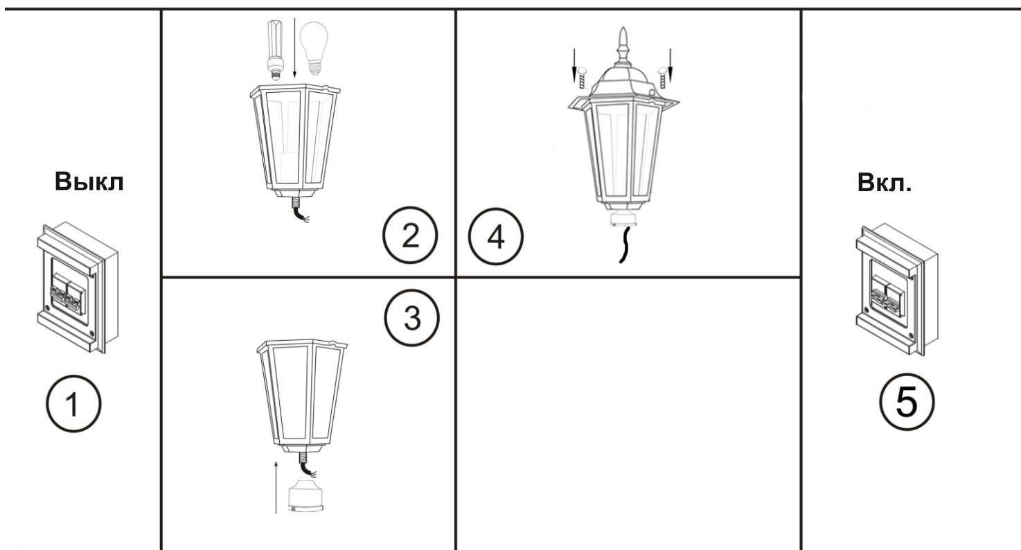
Рис.1. Сборка и установка светильника
