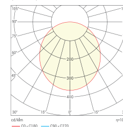
Косинусная КСС (опал)
