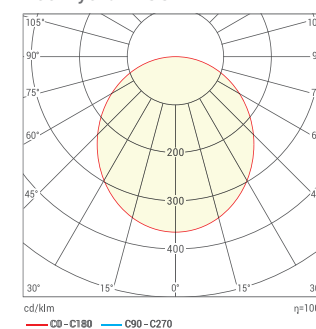
Косинусная КСС
