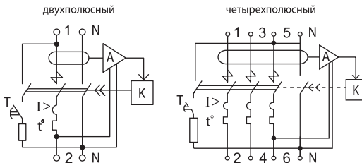
Рисунок 2. Схема подключения
