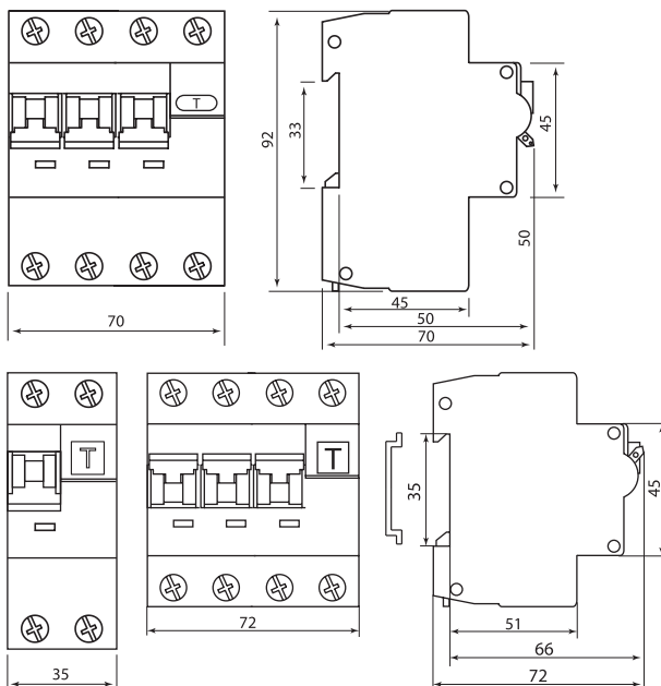
Рисунок 1. Габаритные размеры, мм
