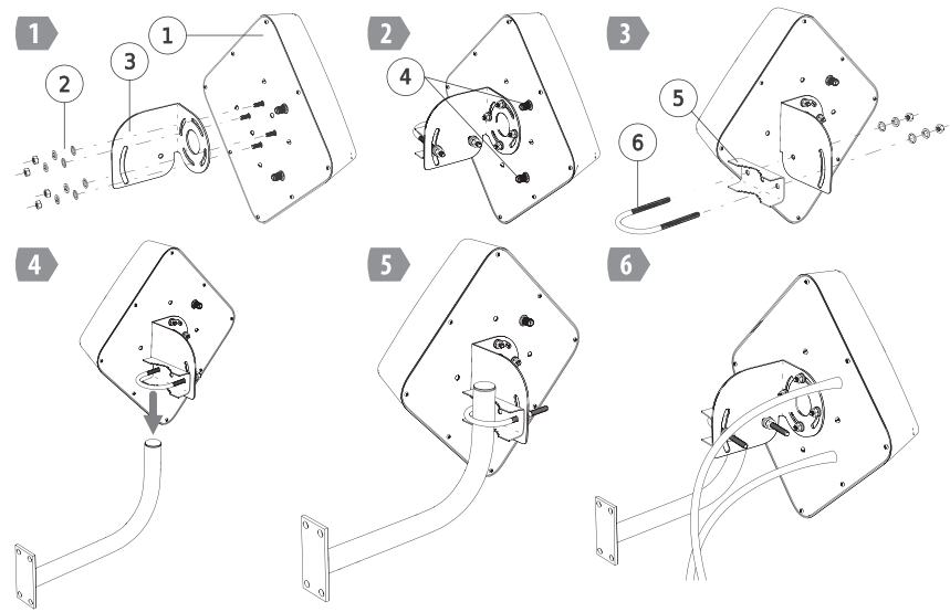
Рисунок 2 – Сборка и монтаж антенны
