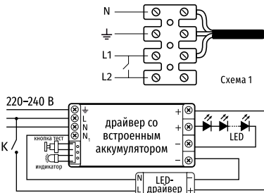
Схема подключения БАП в светильнике ДВО-13-А
