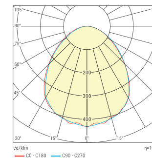
Косинусная КСС (микропризма)
