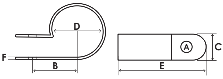
Рисунок 1. Габаритные размеры
