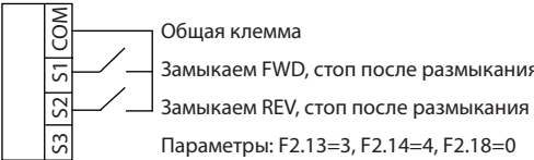
Рисунок 4. Двухпроводная схема управления
