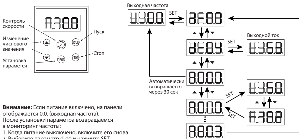
Рисунок 3. Панель преобразователя частоты и программирование
