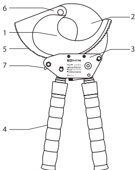
Рисунок 1. Основные узлы секторных ножниц.
