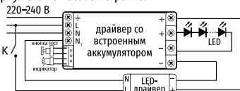
Схема подключения БАП в светильнике ДПБ-01-А
