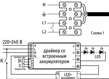
Схема подключения БАП в светильнике ДВО-12-А
