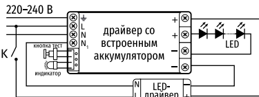
Схема подключения БАП в светильнике ДВО-07-А
