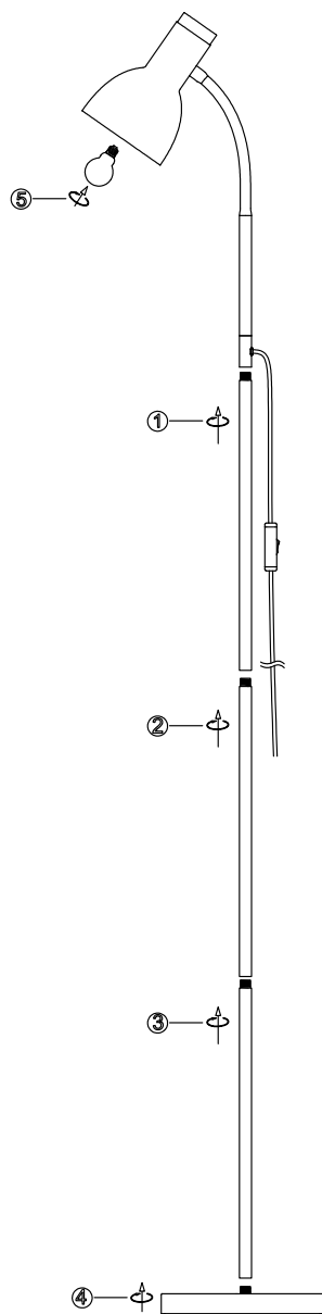
Рис.3, Сборка светильника.
