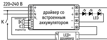
Схема подключения БАП в светильнике ДВО-04-А
