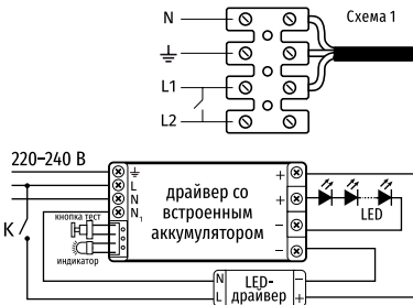
Схема подключения БАП в светильнике ДВО-01-К-А
