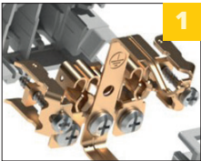
1 токоведущая часть розеток на 16А выполнена из оловянно-фосфорной бронзы
