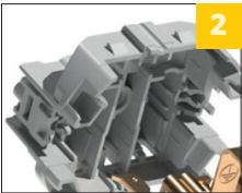
2 внутренний блок из полиамида 6.6
