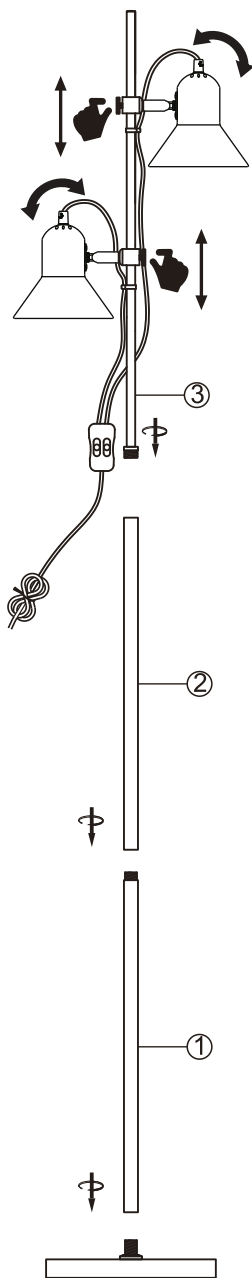
Рис.3, Сборка светильника.
