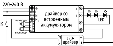
Схема подключения БАП в светильнике ДВО-07-А
