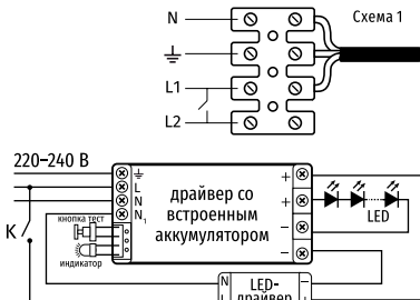
Схема подключения БАП в светильнике ДВО-17-А
