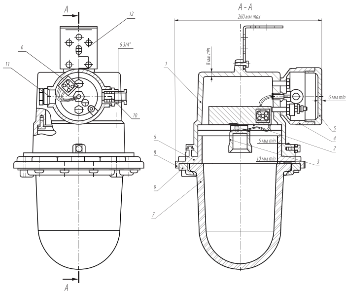
Рисунок 1. Устройство светильника
