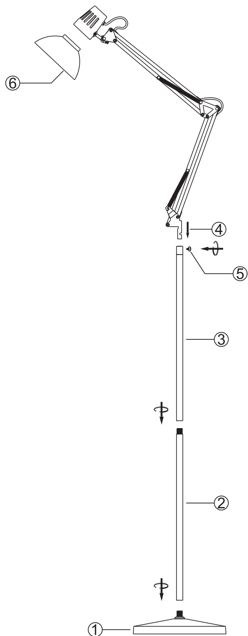
Рис.3, Сборка светильника.
