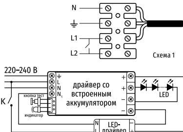
Схема подключения БАП в светильнике DBO-15-A
