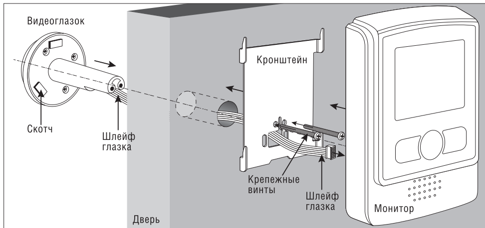
Рисунок 3. Установка видеоглазка
